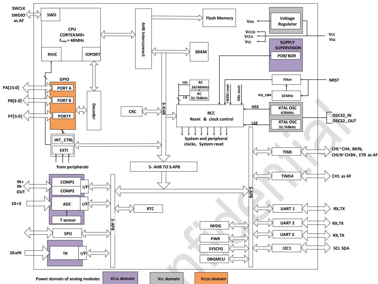
图 1-1 功能模块
